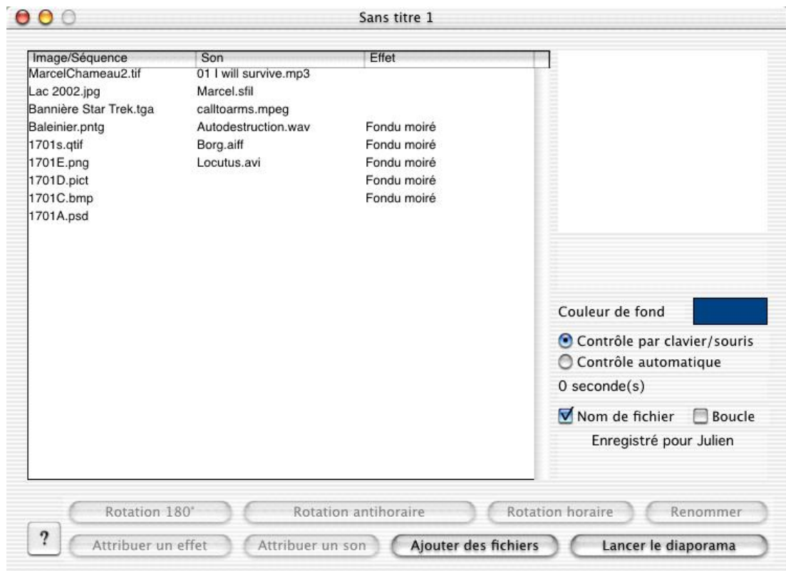
FIG. 3.2 – Copie d'écran
